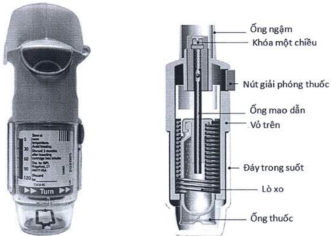
Hình 12: Cấu tạo của Respimat
