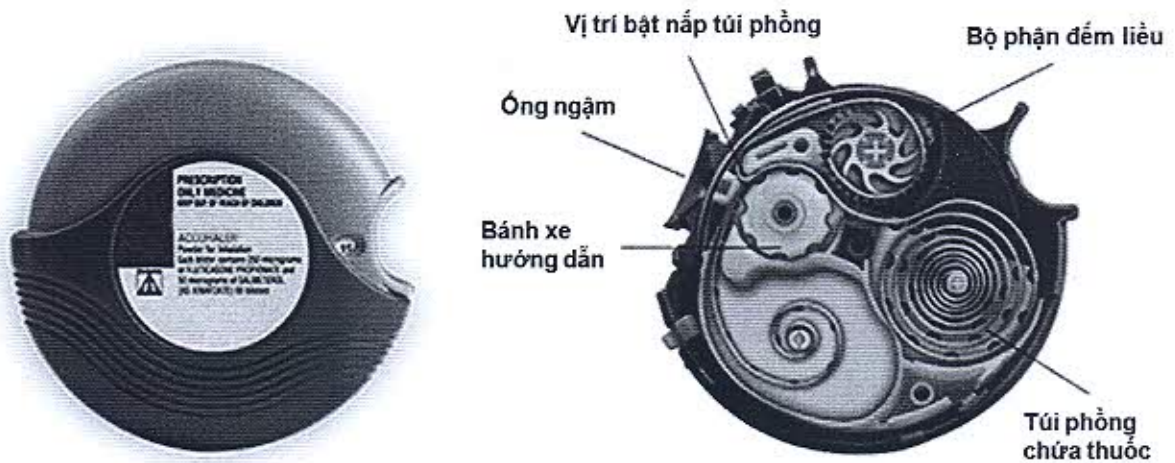
Hình 8: Cấu tạo của Accuhaler
